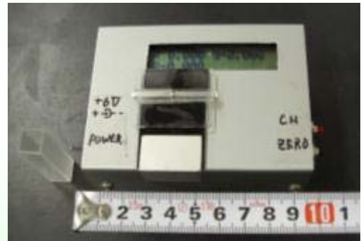
3波長同時測定小型比色計 東京都が公募した「土壤汚染調査における簡易分析法（土壤汚染対策における調査費用の低減化、分析時間の短縮化を図ることを目的として、重金属等を対象に、簡易迅速で優良な13の分析法を選定）」において六価クロムの定量法の一つとして採用。
