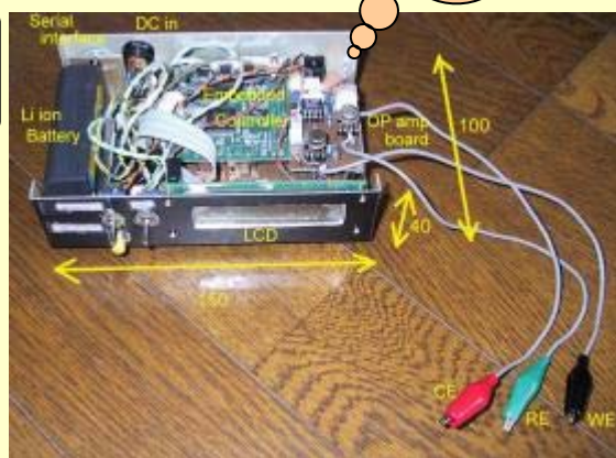
可搬型ポテンショスタット
