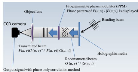
ホログラフィックメモリを用いた 高速画像照合器
